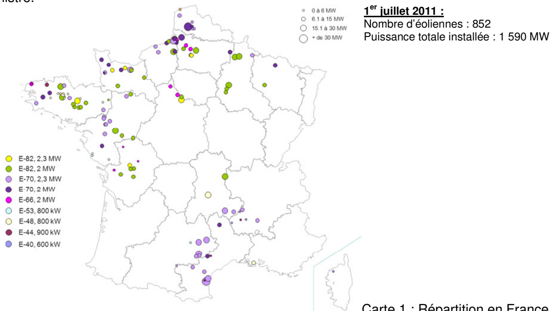
Carte 1 : Répartition en France des parcs éoliens utilisant la technologie ENERCON (Source : ENERCON 2011)
