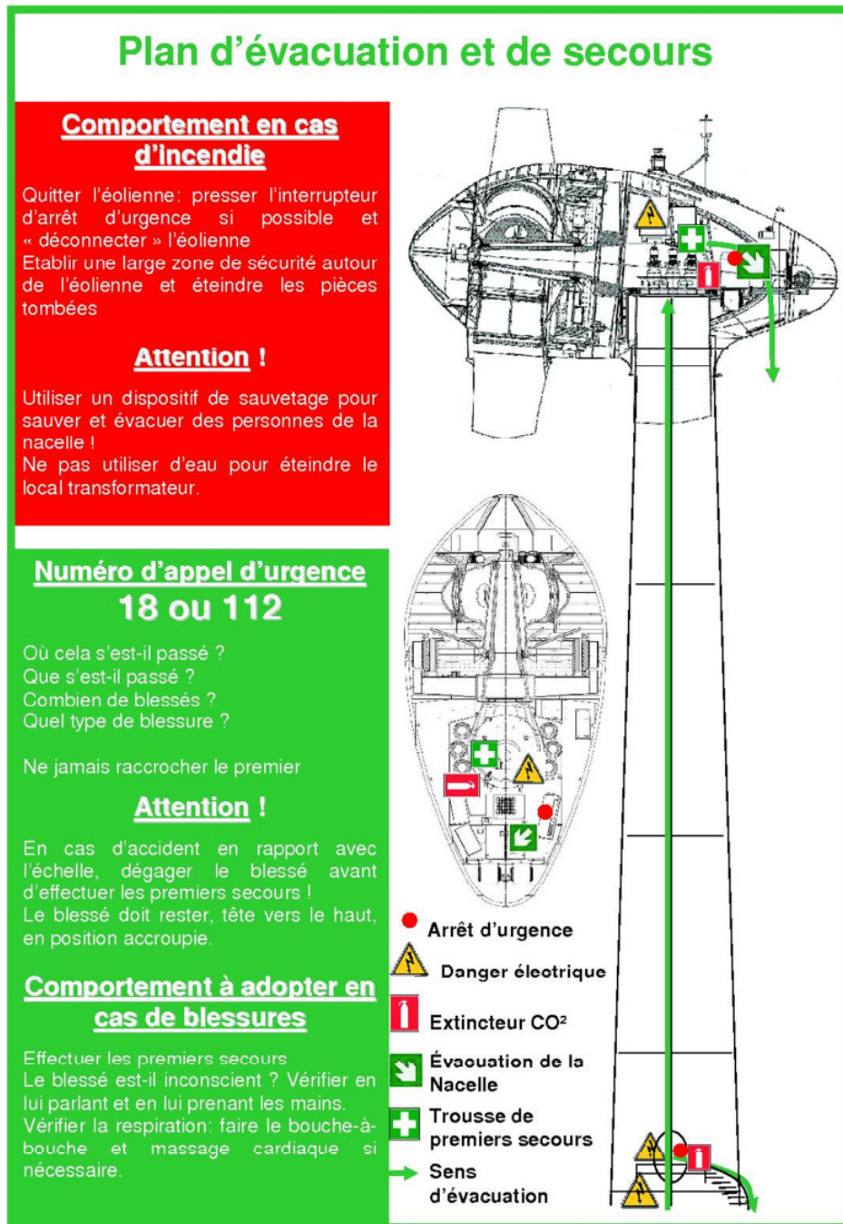
Figure 8 : Plan d'évacuation et de secours dans une éolienne (Source : ENERCON, 2011)
